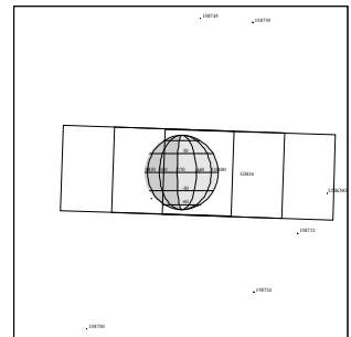
G8ISVOLUND01 GTE-CDS 172:60:0 97-127/13:01:36
