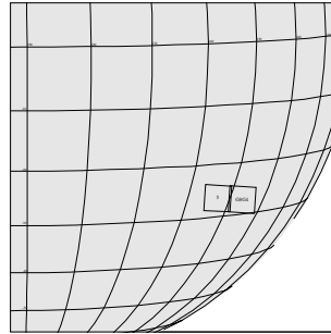
G8GSRNGBAS01 GTE-CDS 50:00:0 97-127/15:05:38
