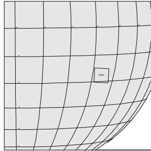
G8GSMARIUS01 GTE-CDS 60:00:0 97-127/14:55:31
