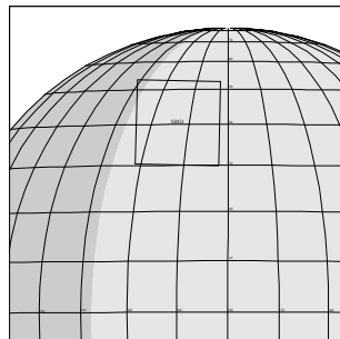
G8GSREGCON01 GTE-CDS 184:60:0 97-127/12:49:28
