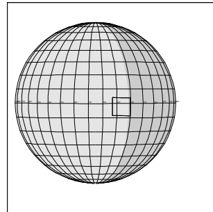
C3ESAJTERM01 EEE+CDS 61:00:0 96-311/19:51:56
