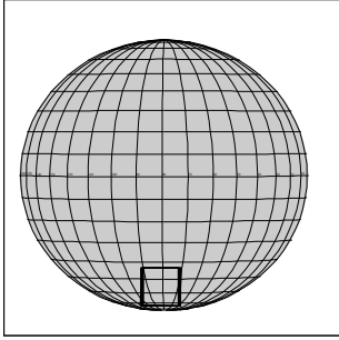
C3JSAURORA03 JOC-CDS 72:45:0 96-314/04:55:03
