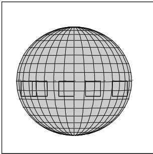
C3JSLTGSCN04 JOC-CDS 54:45:0 96-314/05:13:15
