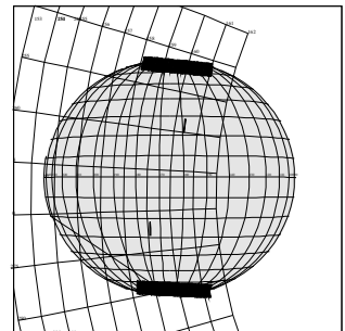
C3JNAURORA01 96-311/05:10:14
