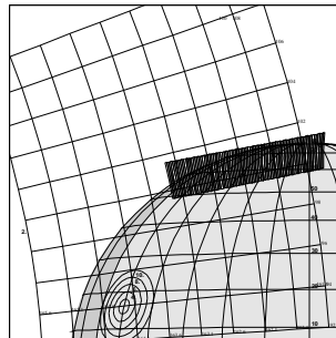
C3JNPFTRAK01 JTB+CDS 528:00:0 96-310/16:49:06
