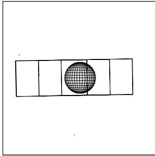
10ISIOGLOC06 97-262/20:39:25
