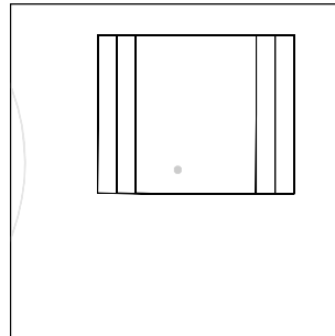
10ESEURPLM02 97-278/21:47:21
