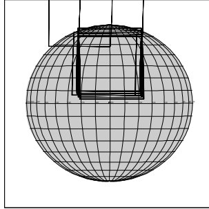
10JSAURORA04 97-279/03:33:09
