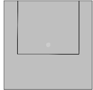
10ISIOAURO01 97-278/21:03:52
