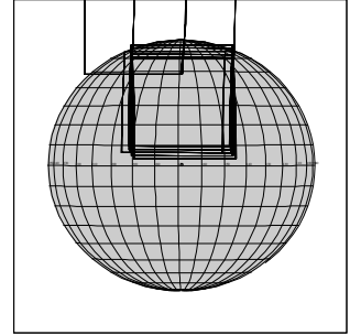
10JSAURORA06 97-279/04:03:29
