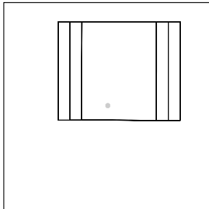
10ESEURPLM01 97-278/21:13:59
