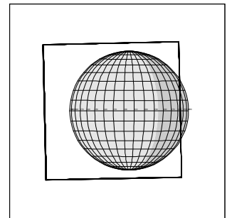
10ISIOGLOC03 IEE+CDS 479:00:0 97-262/12:48:15
