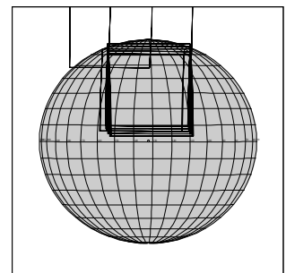
10JSAURORA03 97-279/03:02:49
