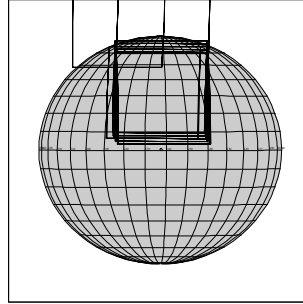
10JSAURORA05 97-279/03:53:22
