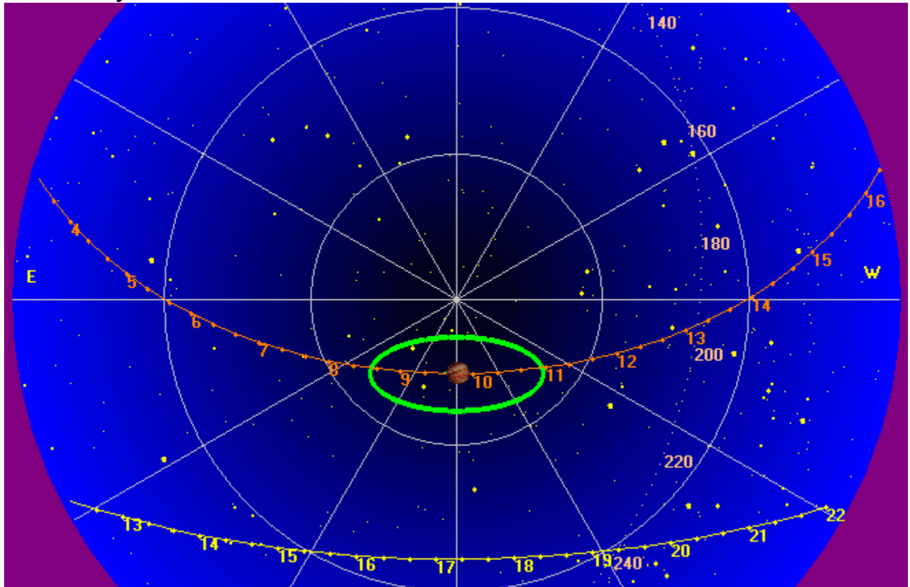
TFD Array 20 MHz HPBW 15° NS x 35° EW
