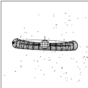
24TU24NANS01 IEE+CDS 1174:00:0 99-285/00:20:00
