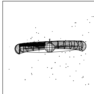
24TU24NANS02 99-285/05:33:26
