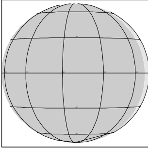
24JPWAVEST01 99-283/09:01:04
