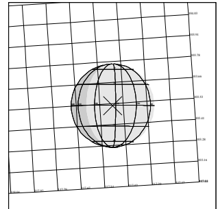
15IUHRSPEC01 98-151/18:50:21
