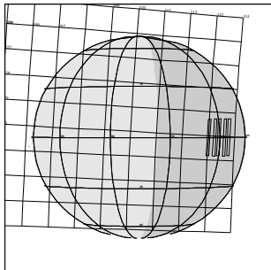
15JUDARKSIDE 98-152/19:49:50
