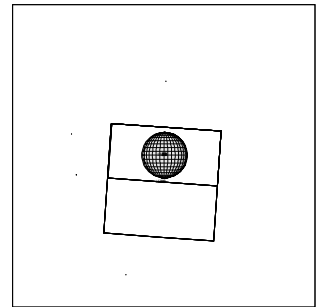
15ISECLIPS03 98-152/18:43:06
