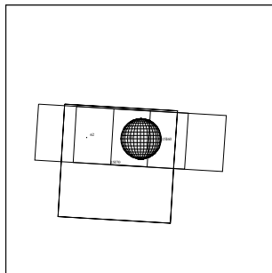
15ISKANEHI01 98-152/21:14:46
