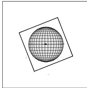
15ISSRFMON01 98-152/08:57:40
