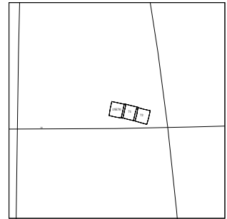
15ESRELIEF01 98-151/21:08:53
