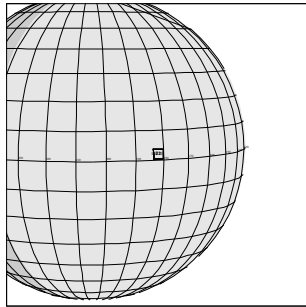
15ESCILIXS01 98-151/20:38:33
