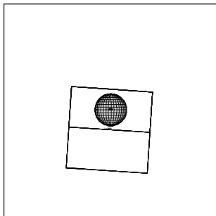
15ISECLIPS04 98-152/19:35:41
