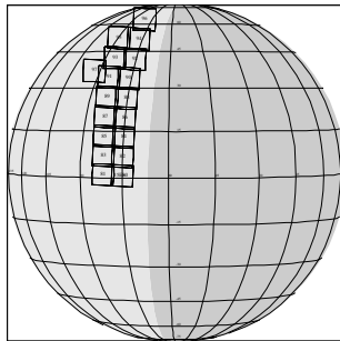
15ESREGMAP02 98-151/22:11:34
