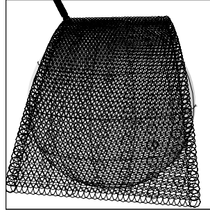
25EPDGTM_01 EEE+CDS 60:00:0 99-329/17:29:32
