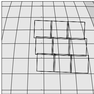
14ESTYREHR01 EEE+CDS 41:00:0 98-088/14:02:19
