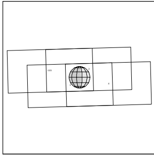
11ISECLIPS01 IEE-CDS 4265:00:0 97-308/23:53:25
