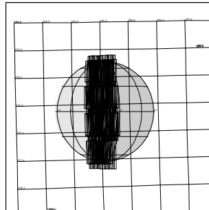
C9GNGLOBAL02 97-177/21:54:17
